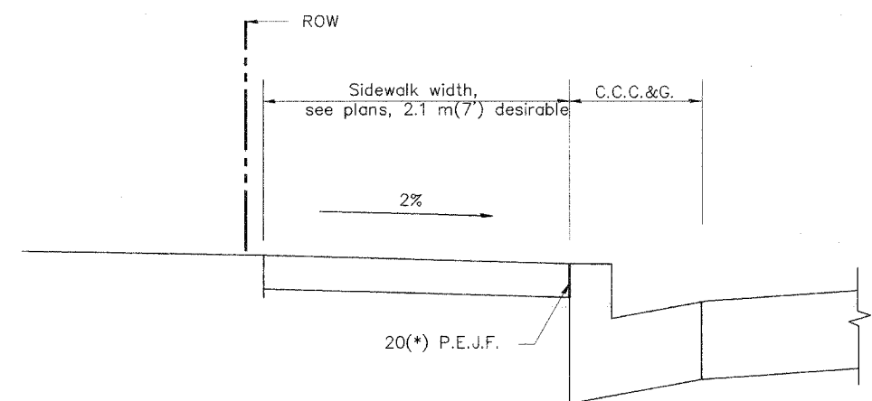
SECTION D-D
