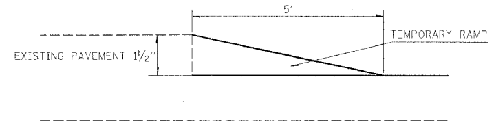
TEMPORARY RAMP DETAIL STA 1141+07 TO STA 1141+12 STA 19+42 TO STA 19+47
