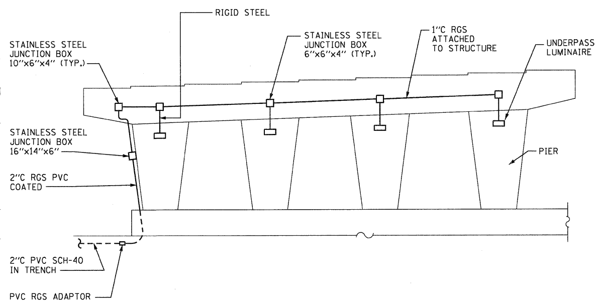
UNDERPASS LUMINAIRE MOUNTING DETAIL SCALE: N.T.S.
