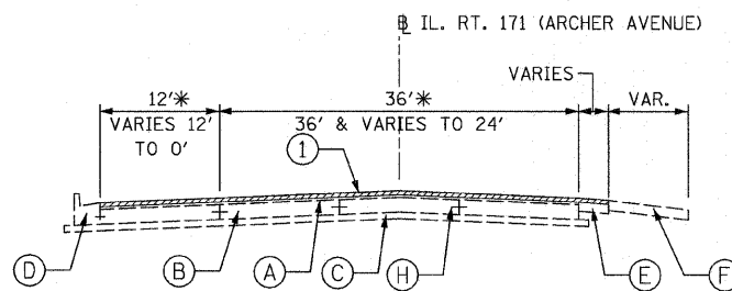
EXISTING TYPICAL SECTION * STA. 17+75 TO STA. 25+10 STA. 97+00 TO STA. 100+90
