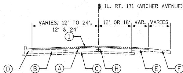
EXISTING TYPICAL SECTION STA. 124+50 TO STA. 127+10 STA. 181+50 TO STA. 183+00 STA. 254+00 TO STA. 261+32 STA. 261+32 TO STA. 272+55 - PAVING OMISSION
