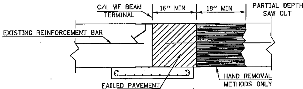
SECTION D-D
