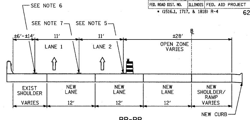
RR-RR STAGE 3A: NB I-57; STA. 191+42 TO STA. 205+07
