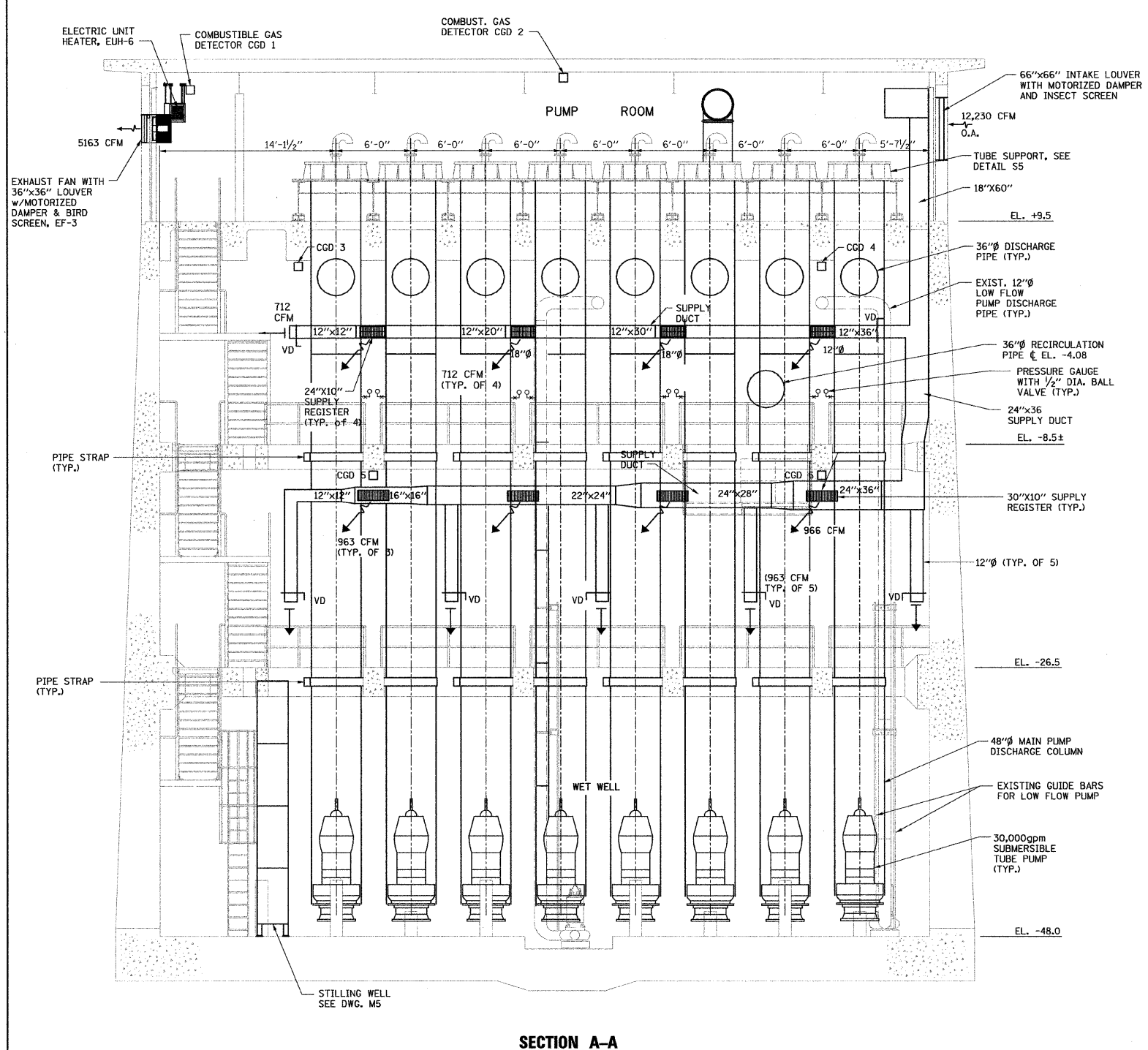
SECTION A-A
