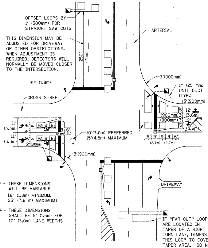
DETAIL 2 N.T.S.
