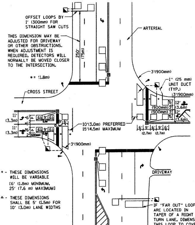
DETAIL 2 N.T.S.
