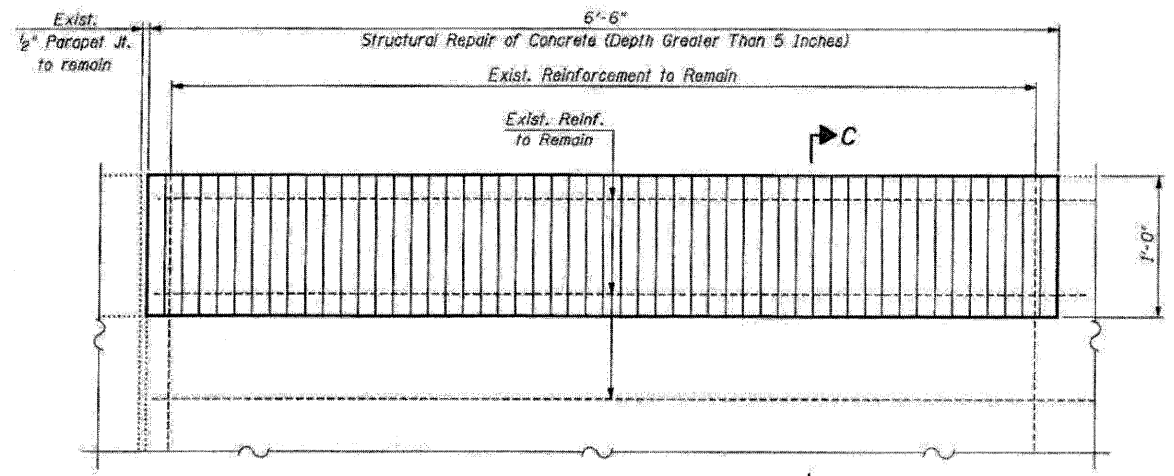
DECK PLAN (Scale: Not to Scale)
