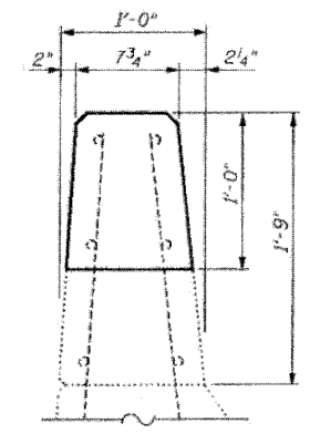
SECTION C-C (Scale: Not to Scale)
