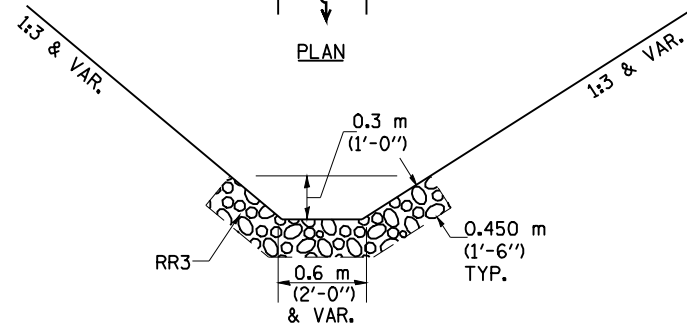
ELEVATION OPTION 2
