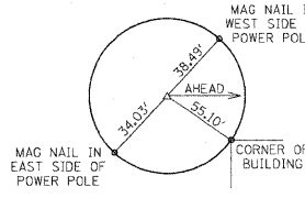
POT STA 0+00.00 (ALLEY @ STA 149+27.00) = ML STA 149+27.00 (MAG NAIL)
