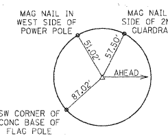
POT STA 0+00.00 (CHEROKEE DR.) = ML STA 108+46.00 (MAG NAIL)
