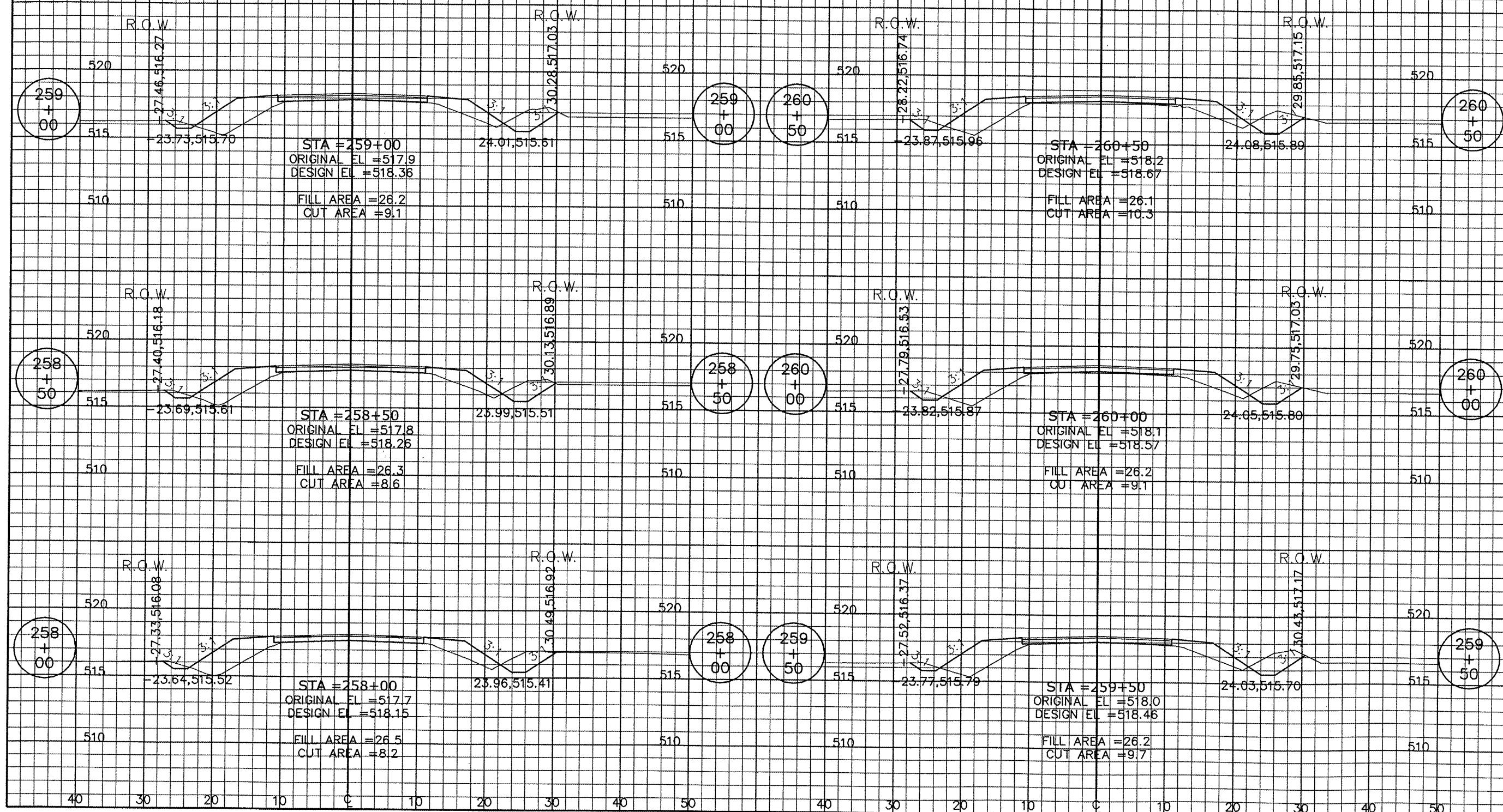
CROSS SECTIONS STA. 258+00 TO STA. 260+50
