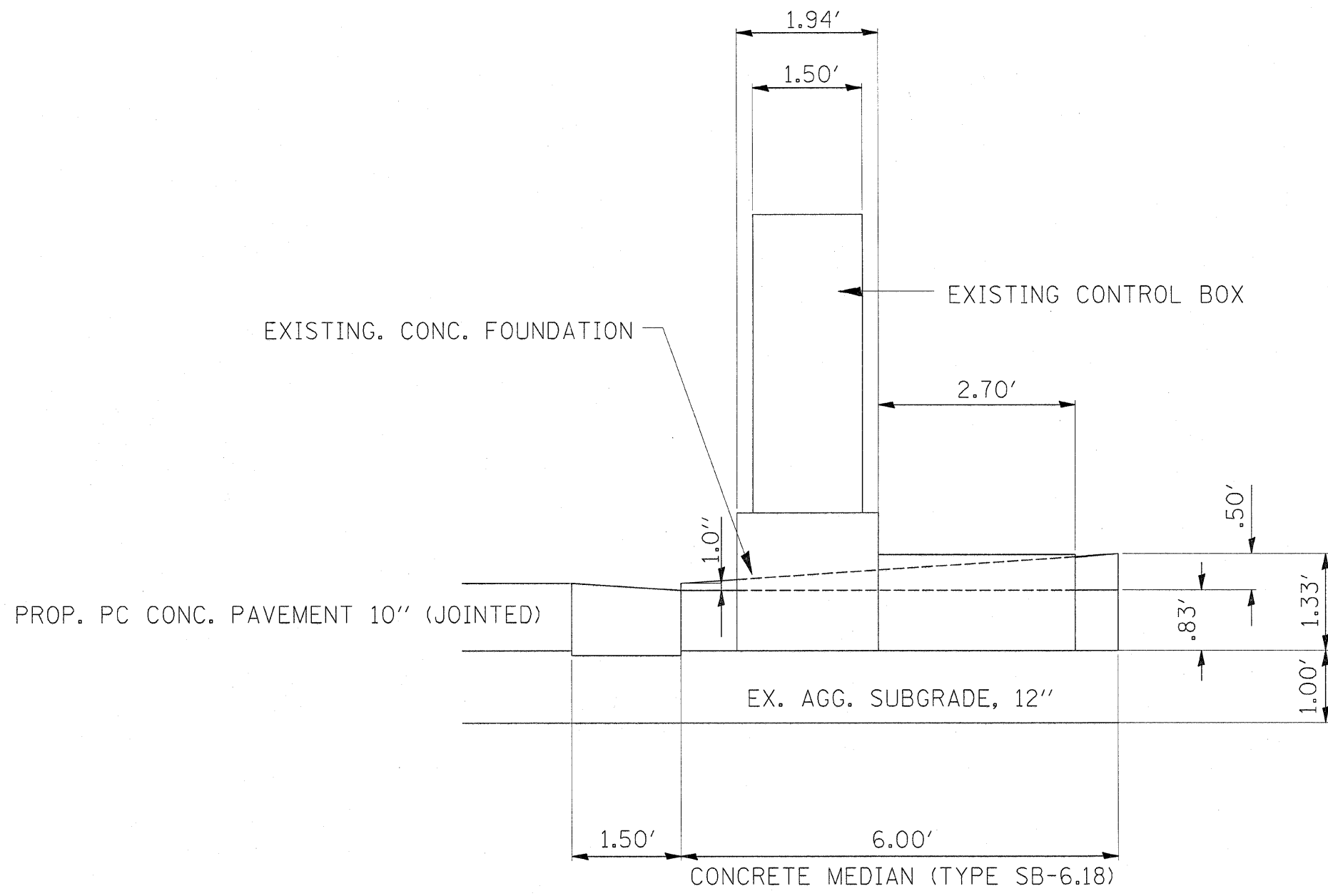
SECTION A-A
