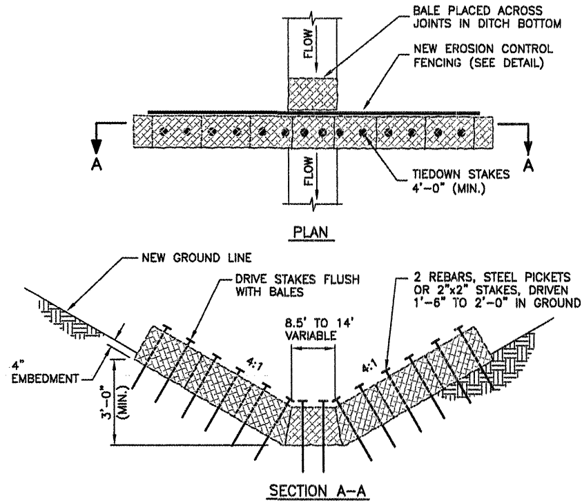
TEMPORARY DITCH CHECK N.T.S.
