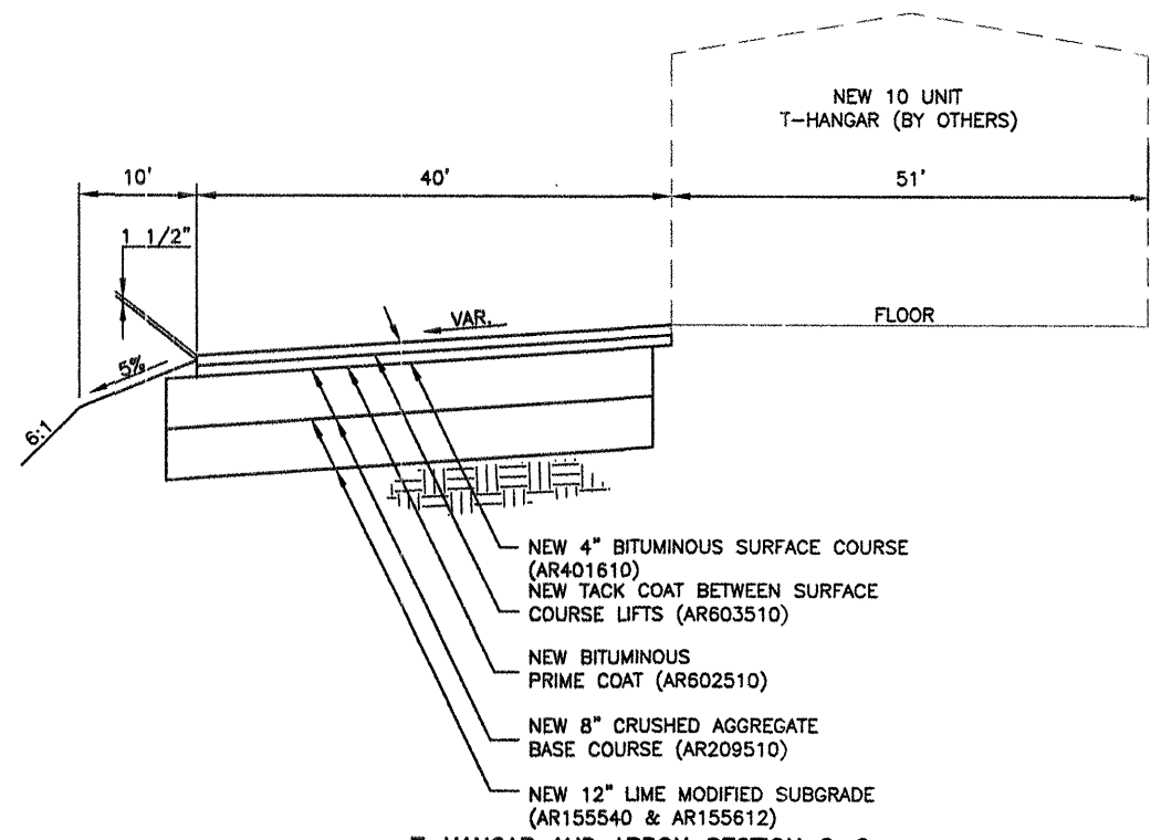
T-HANGAR AND APRON SECTION C-C N.T.S.
