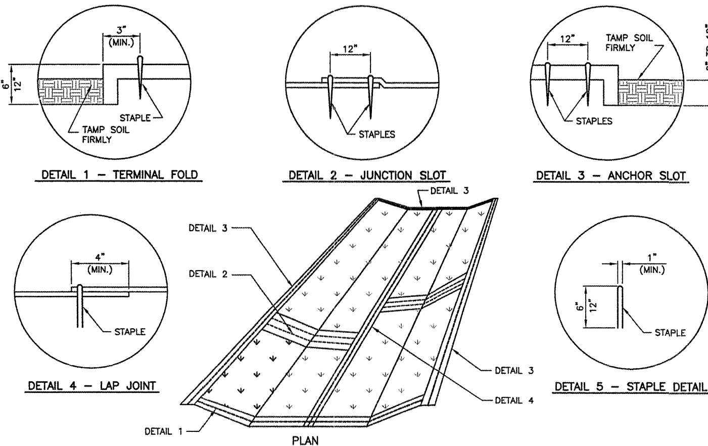
EXCELSIOR BLANKET DETAILS N.T.S.
