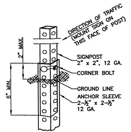
POST TYPE N.T.S.
