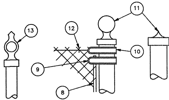
PEDESTRIAN GATE DETAIL N.T.S.
