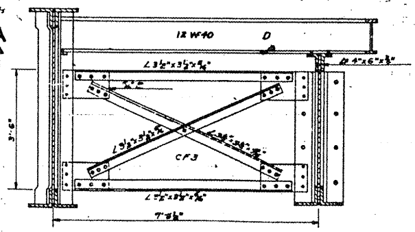
SEC. A-A
