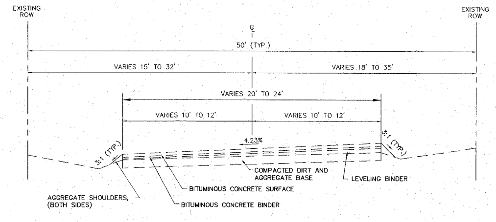
EXISTING TYPICAL SECTION STA 78+43 TO STA 82+48
