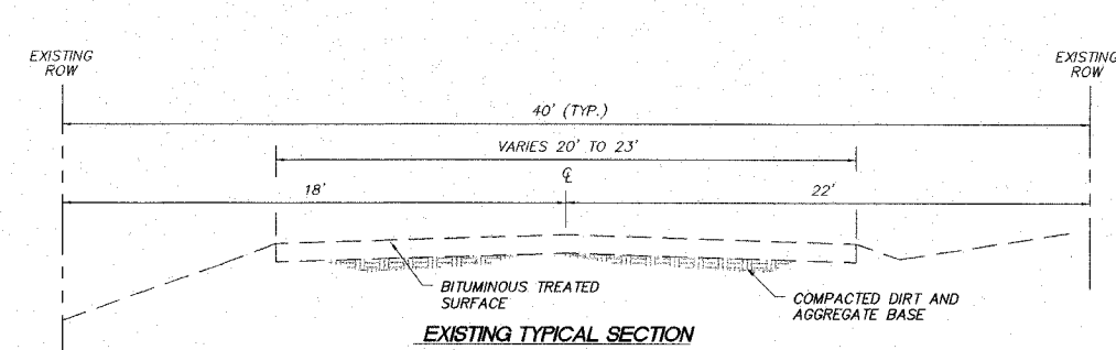
EXISTING TYPICAL SECTION STA 78+43 TO STA 82+48
