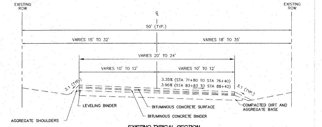
EXISTING TYPICAL SECTION STA 71+80 TO STA 76+40 STA 83+83 TO STA 88+42
