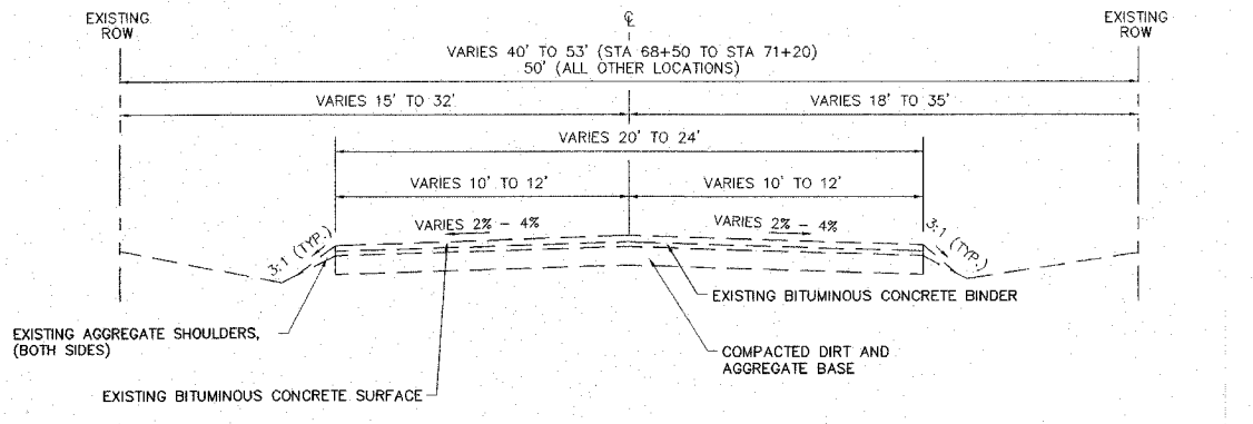
EXISTING TYPICAL SECTION STA 68+50 TO STA 71+80 STA 76+40 TO STA 78+43 *STA 82+48 TO STA 83+83 STA 88+42 TO STA 88+83
