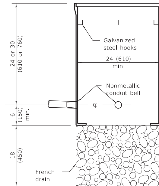
ELEVATION
