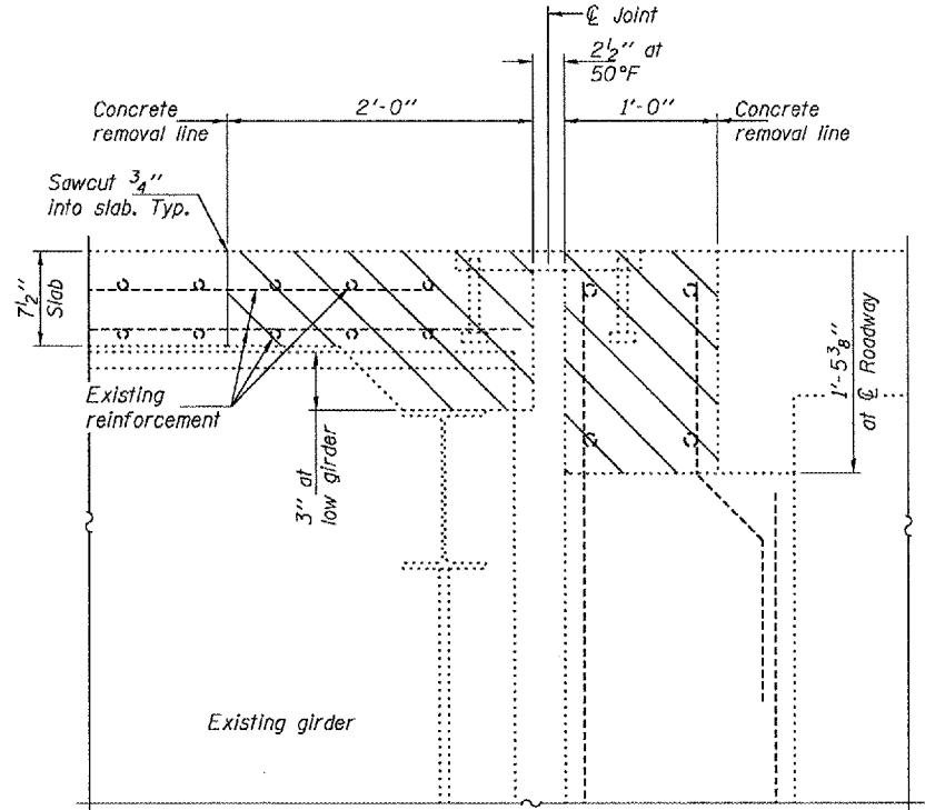
SECTION A-A
