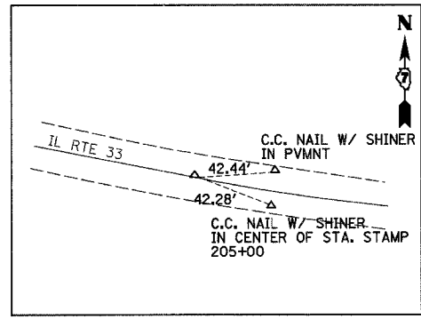
P.T. STA. 204+70.94 (MAG NAIL)
