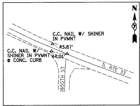
P.C. STA. 197+48.45 (MAG NAIL)
