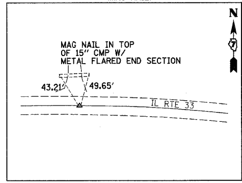
P.C. STA. 339+25.07 (MAG NAIL)
