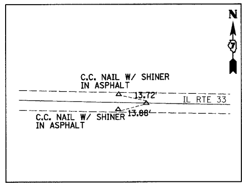
P.C. STA. 323+04.51 (MAG NAIL)
