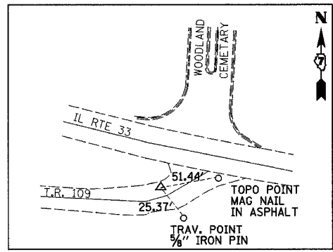
P.I. STA. 201+14.06 (5/8" IRON PIN)
