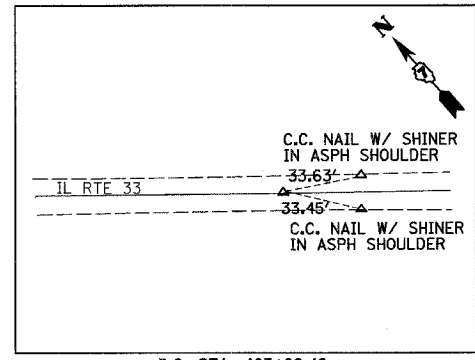
P.C. STA. 463+69.48 (MAG NAIL)
