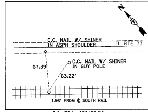
P.I. STA. 477+99.84 (5/8" IRON PIN)
