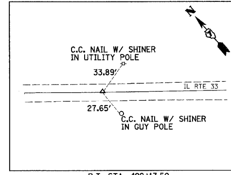
P.T. STA. 492+17.50 (MAG NAIL)
