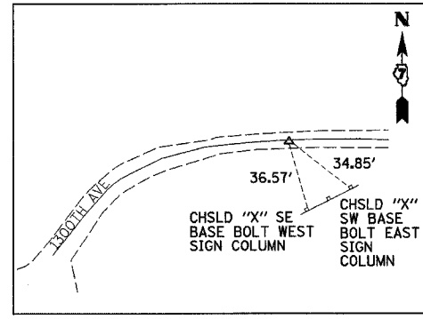
P.I. STA. 347+72.53 (MAG NAIL)
