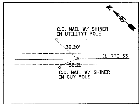
P.C. STA. 390+16.07 (MAG NAIL)
