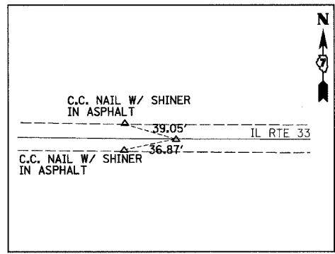
P.I. STA. 326+34.68 (MAG NAIL)
