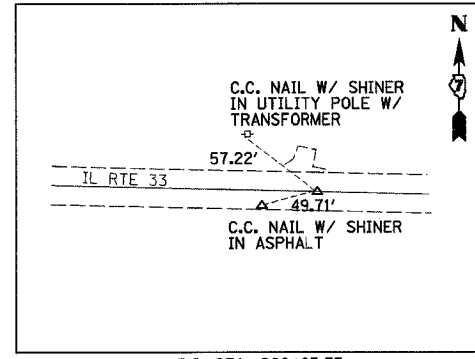
P.I. STA. 260+95.33 (MAG NAIL)
