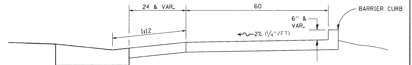
SECTION A-A
