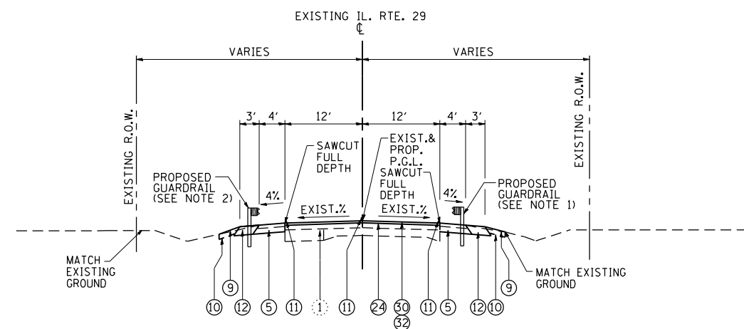
TYPICAL NO. 2 EXISTING IL 29: STA. 151+35.21 TO STA. 153+90.12
