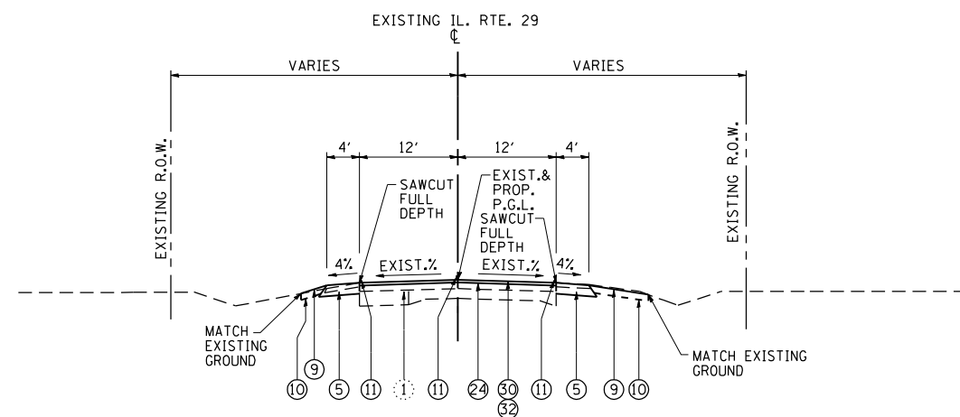
TYPICAL NO. 1 EXISTING IL 29: STA. 89+07.26 TO STA. 151+35.21 STA. 153+90.12 TO STA. 183+96.28
