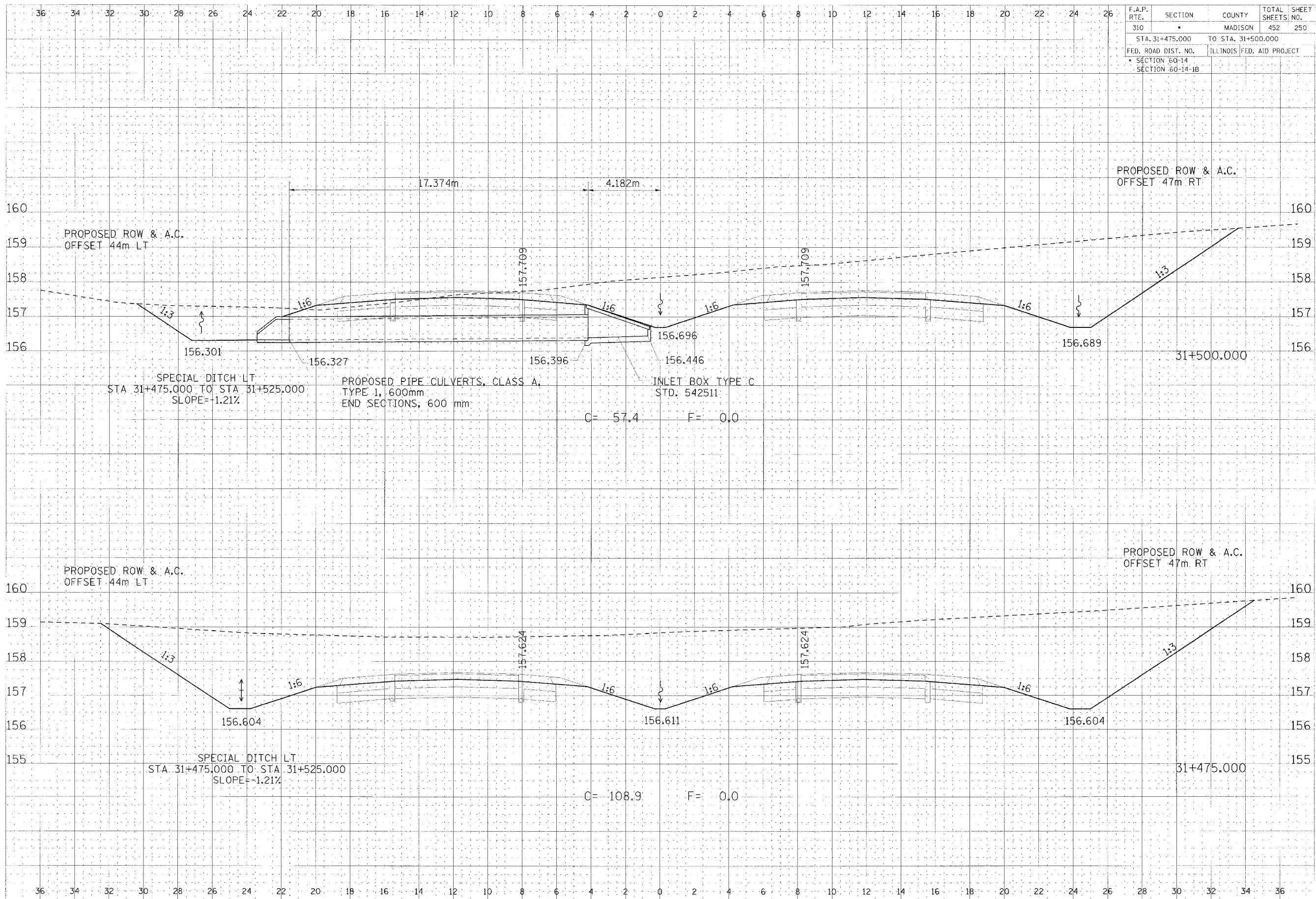
CROSS SECTION, FAP ROUTE 310, STA 31+475.000 TO STA 31+500.000
