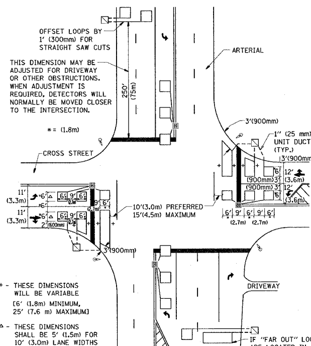
DETAIL 2 N.T.S.
