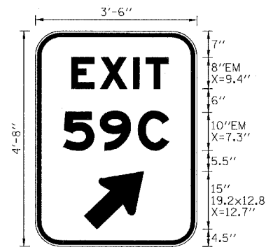
STA. 2348+44
