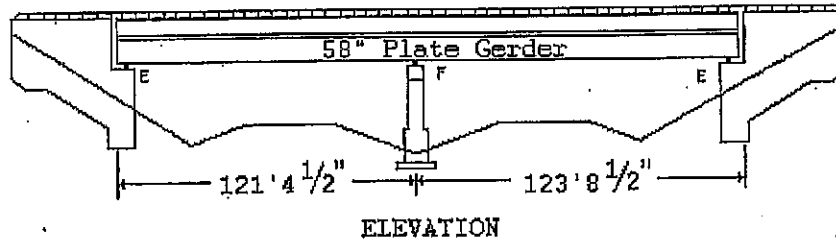
ELEVATION
