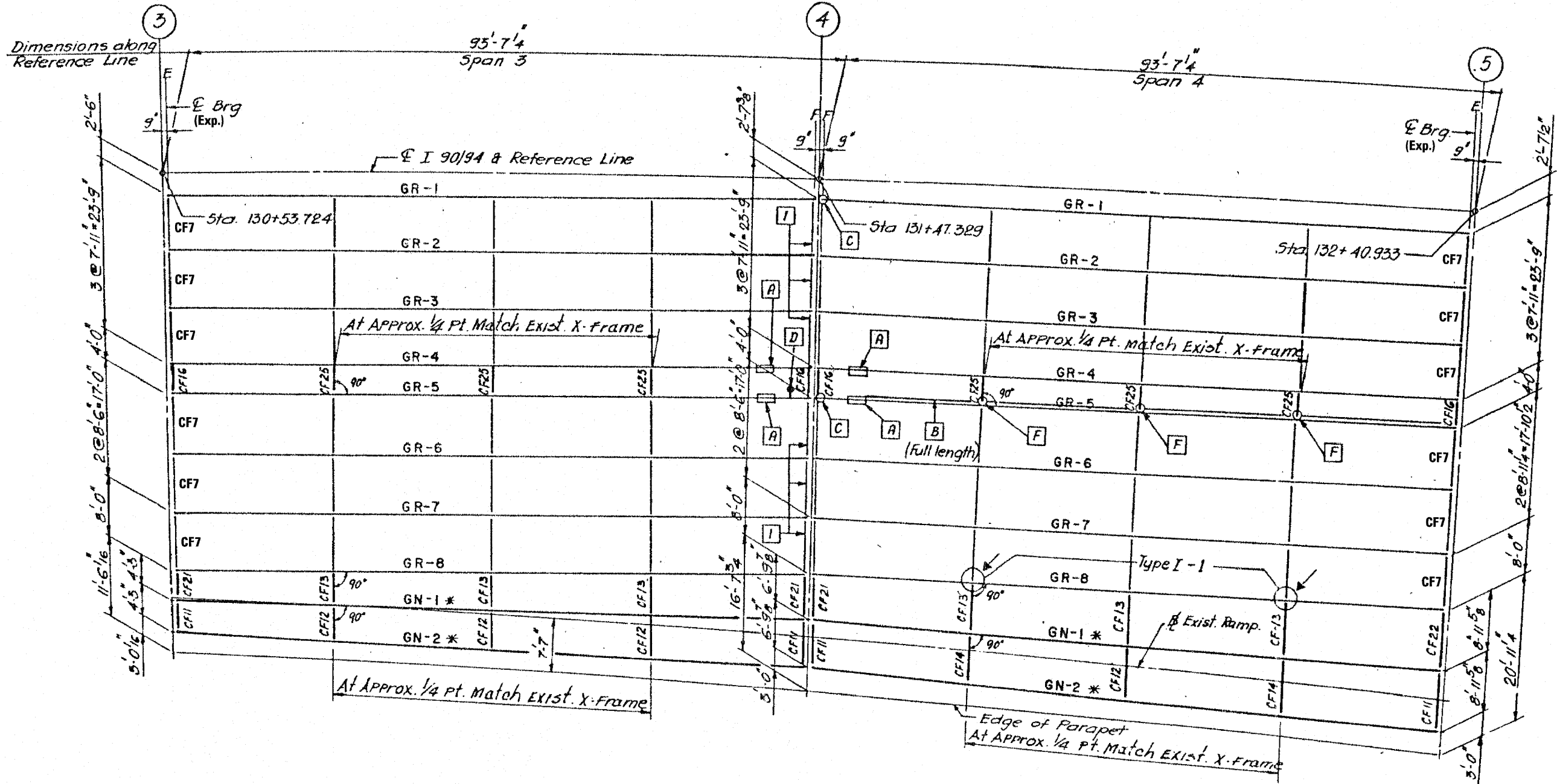
PLAN - SPANS 3 & 4 (N.B.)
