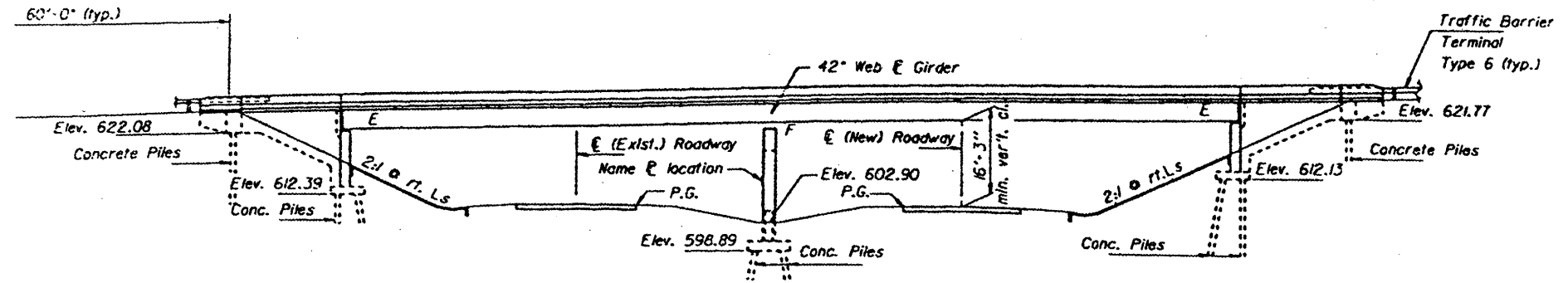
ELEVATION
