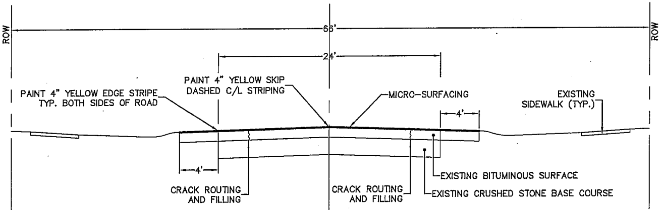
OGDEN AV. - N. COLLEGE AV. TO END STA. 124+00 TO STA. 135+00 SEGMENT "A" N.T.S.
