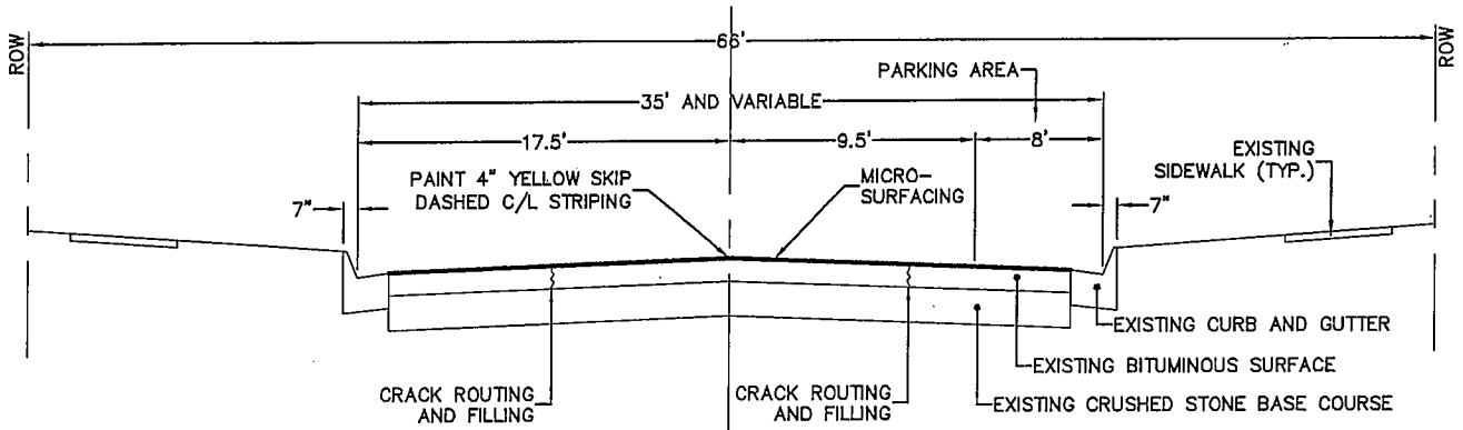
OGDEN AV. - N. COLLEGE AV. TO END STA. 100+00 TO STA. 124+00 SEGMENT "A" N.T.S.
