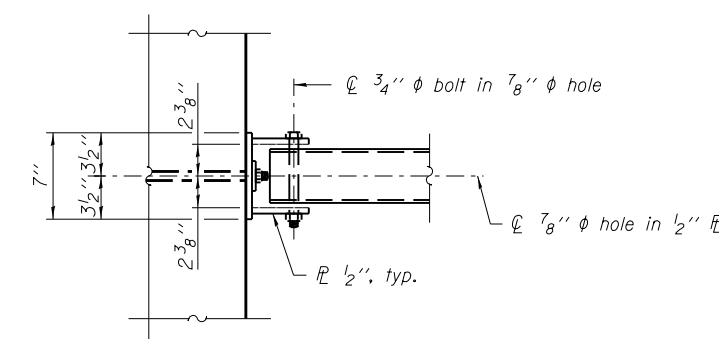
VIEW A-A
