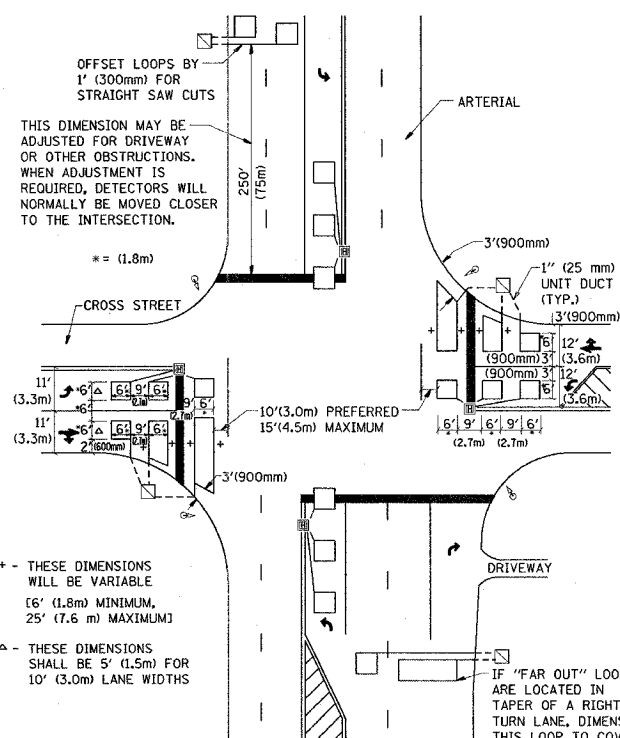
DETAIL 2 N.T.S.
