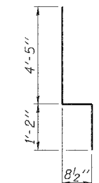
BAR d5(E)
