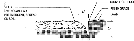
2 SPADED EDGE SCALE: N.T.S.
