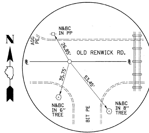
P.T. STA. 46+47.75 OLD RENWICK RD. N. 9700.422, E. 6320.611 (PK NAIL)
