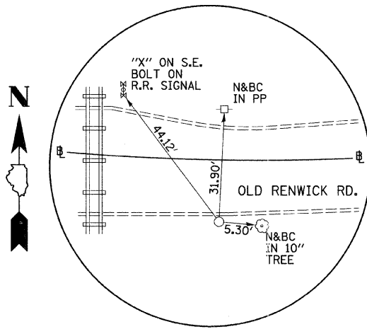
P.I. STA. 44+98.21 OLD RENWICK RD. N. 9589.962, E. 6431.243 (I-ROD)
