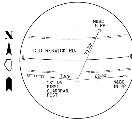
P.I. STA. 39+77.63 OLD RENWICK RD. N. 9447.130, E. 6937.780 (I-ROD)
