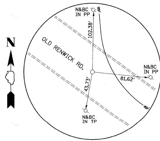
P.I. STA. 49+08.71 OLD RENWICK RD. N. 9884.808, E. 6135.937 (MAG NAIL)
