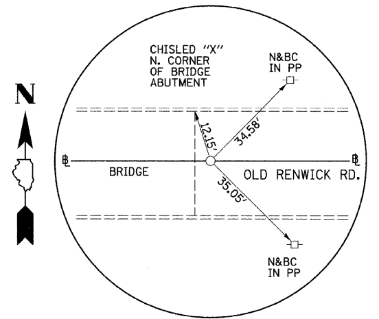
P.T. STA. 40+74.30 OLD RENWICK RD. N. 9474.915, E. 6839.243 (PK NAIL)
