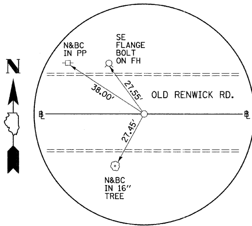
P.C. STA. 38+75.25 OLD RENWICK RD. N. 9477.592, E. 7035.524 (PK NAIL)
