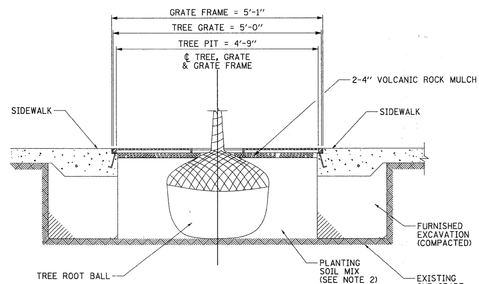
TREE PIT - LONGITUDINAL SECTION N.T.S.
