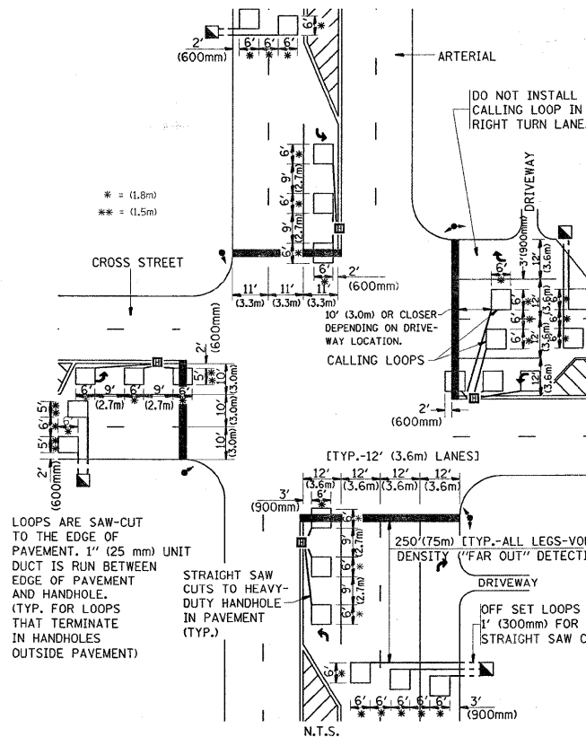
DETAIL 1 N.T.S.
