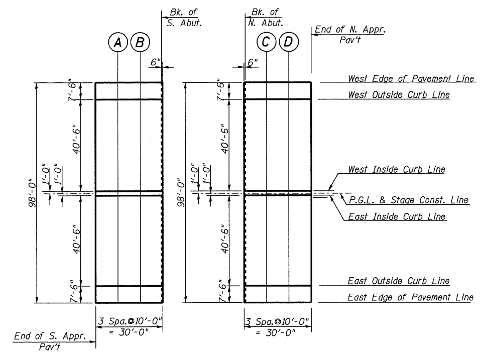
PLAN (S. APPR. PAV'T)
