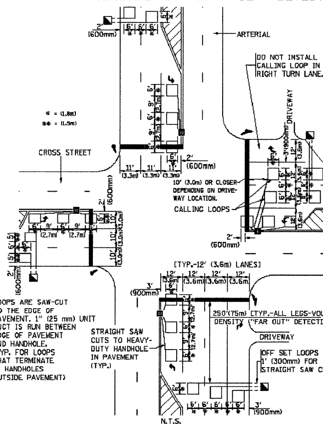
DETAIL 1 N.T.S.
