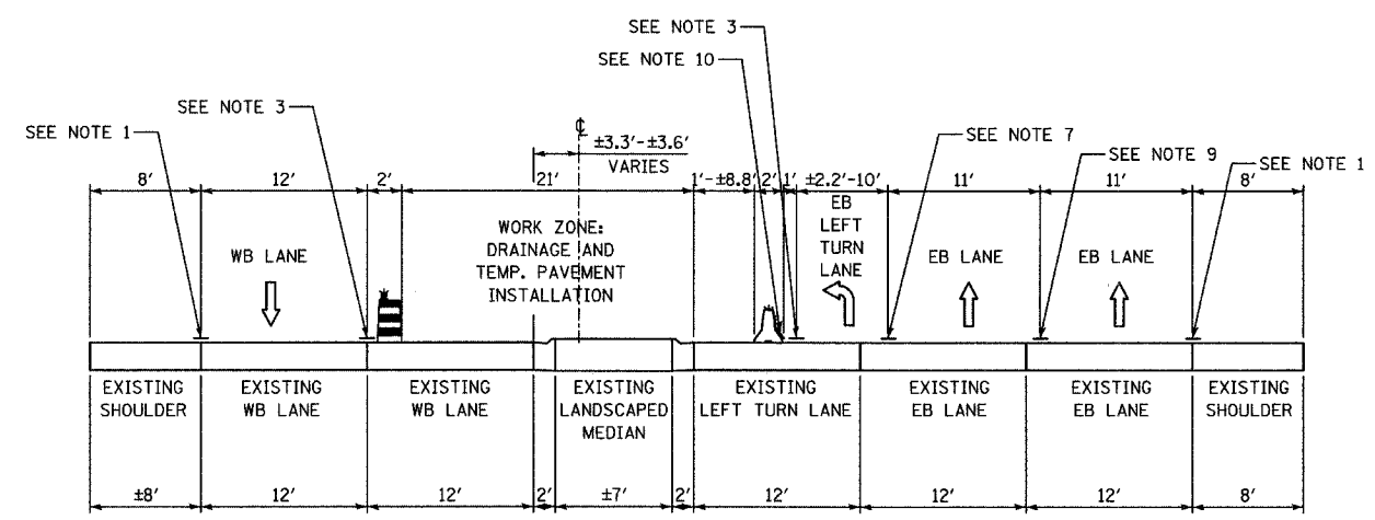
B-B PRE STAGE A: W. 75TH STREET; STA. 146+10 TO STA. 147+50
