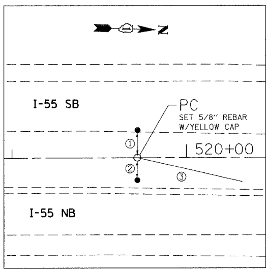
PC STA. 519+71.86
