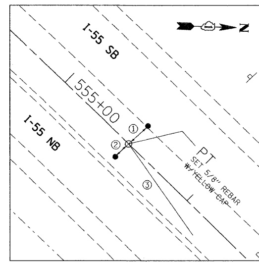
PT STA. 555+51.97
