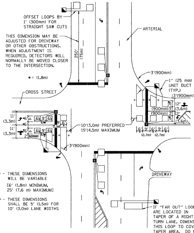
DETAIL 2 N.T.S.
