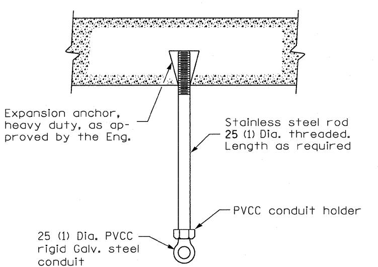
CONDUIT HANGER
