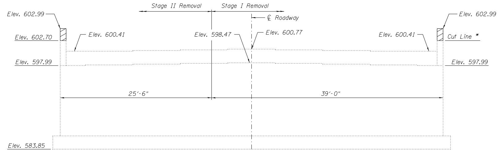
ELEVATION (N. Abut. Shown, S. Abut. Similar)
