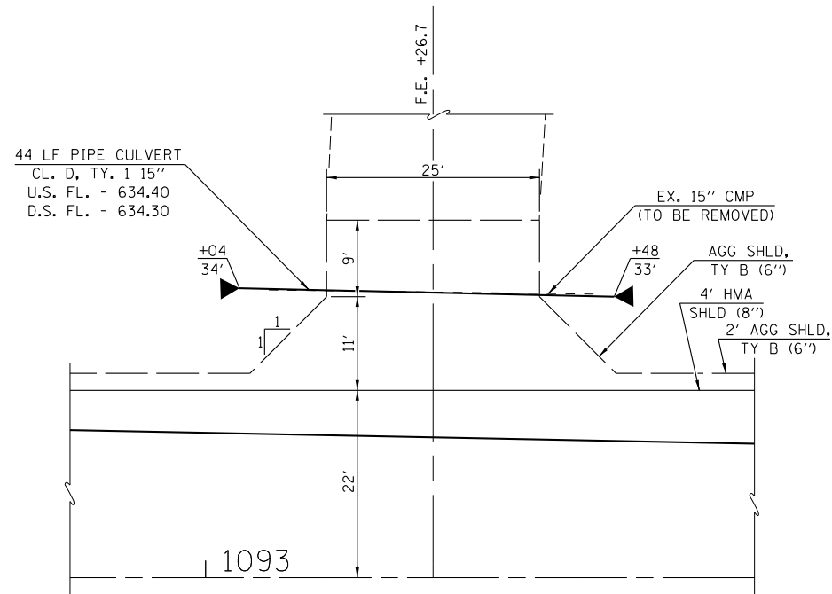
DETAIL (F.E. 1093+26.7)
