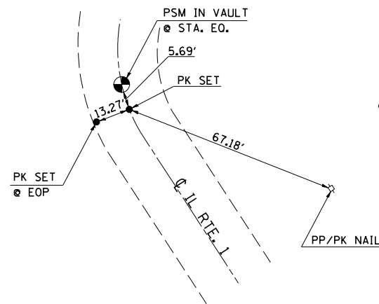
PC 174+77.78 #15 STA. EO. 174+83.42 BK = 175+02.84 AH
