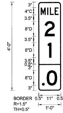
EB-MM-43 STA. 748+20
