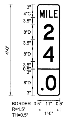
EB-MM-49 STA. 906+60
