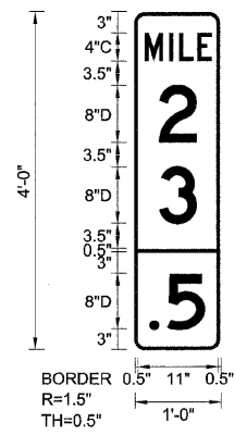
EB-MM-48 STA. 880+20
