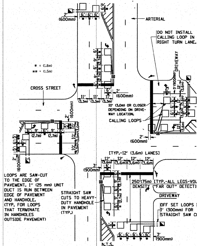
DETAIL 1 N.T.S.
