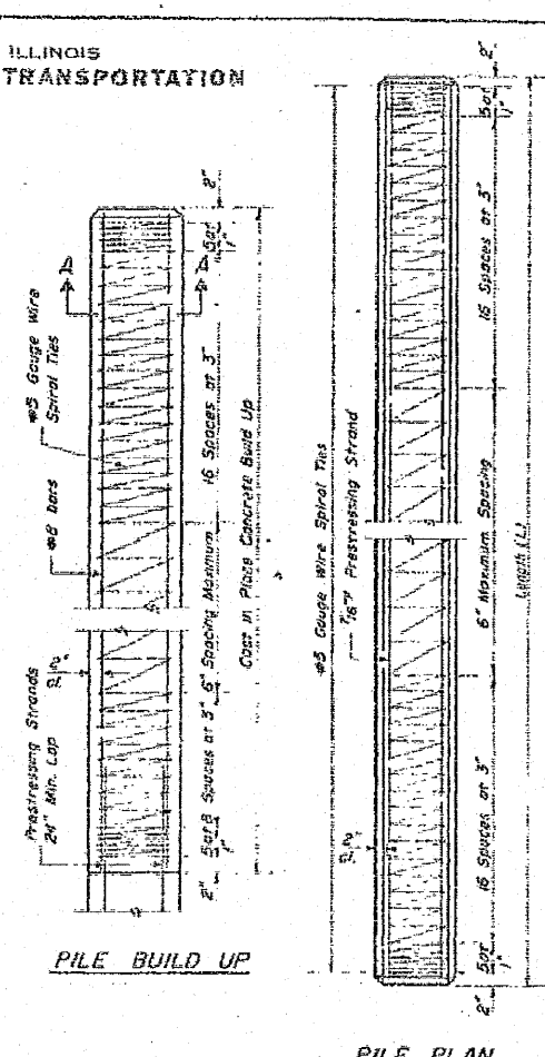
PILE PLAN
