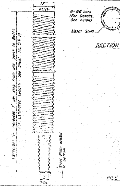
PILE PLAN
