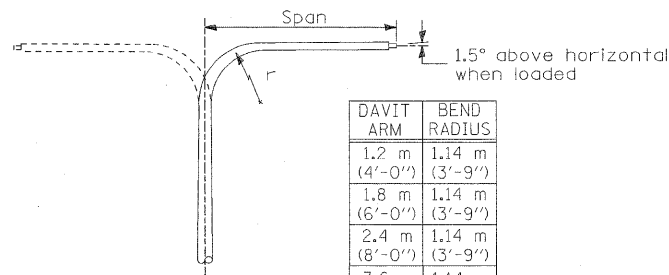
DAVIT ARM
